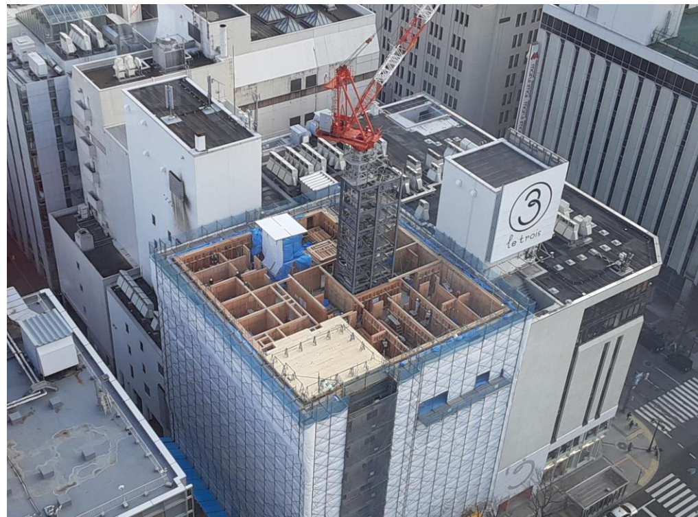
木造ハイブリット枠組工法 施工
